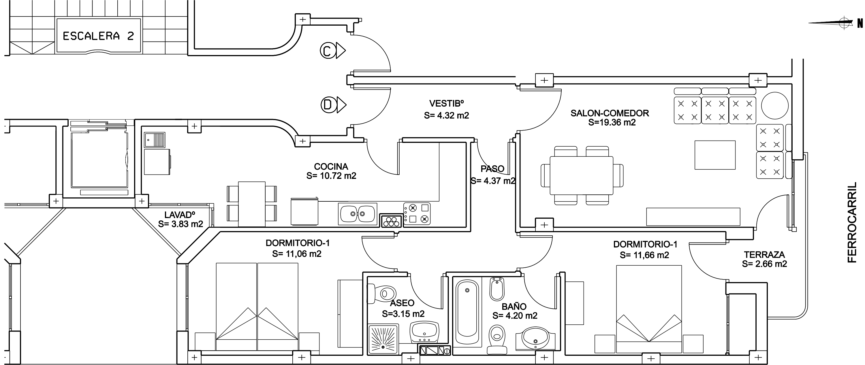
VIVIENDA D ( PLANTAS 1ª y 2ª )
